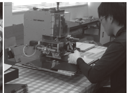
箔押機
